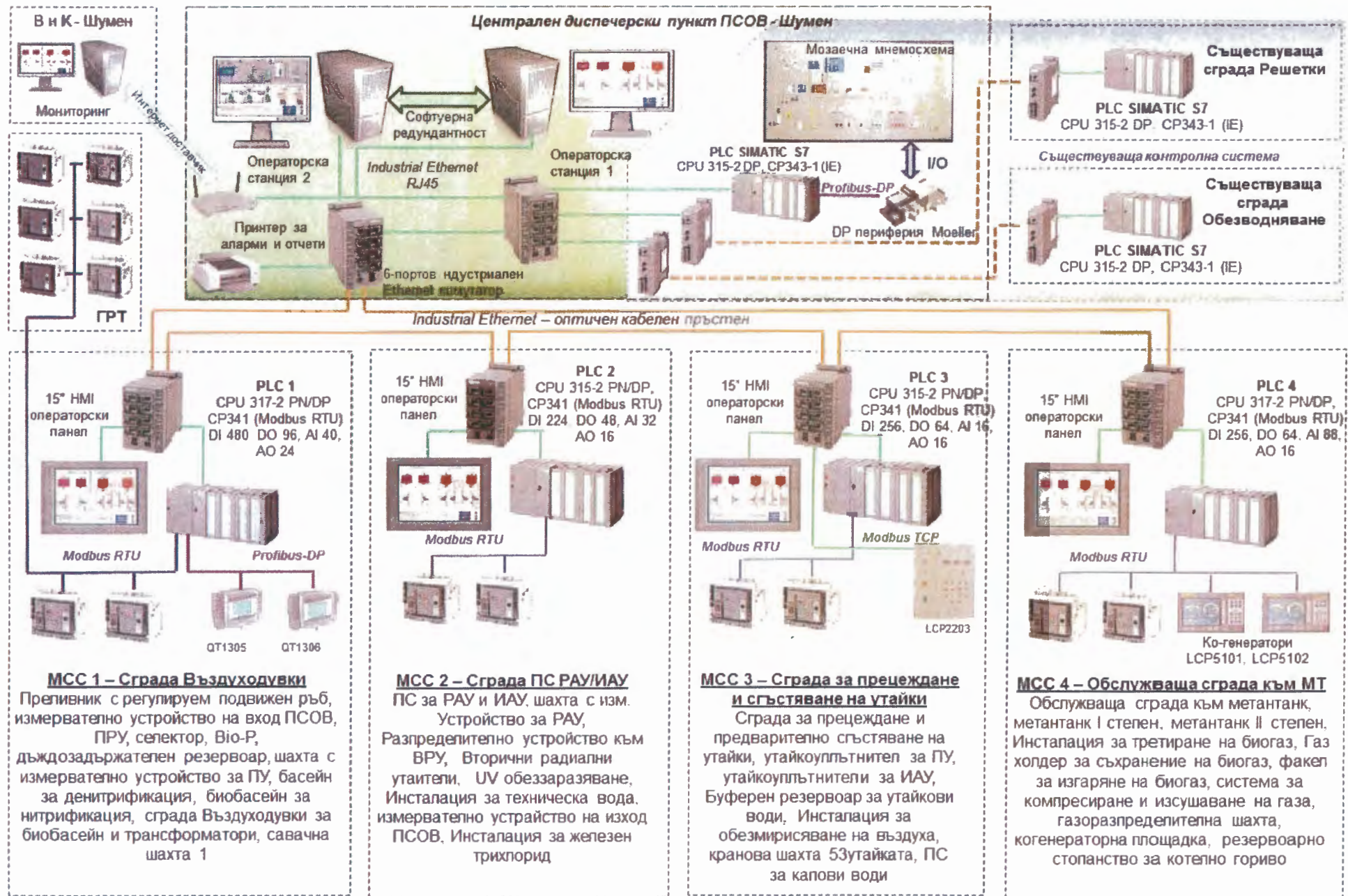
Структура на SCADA системата на ПСОВ „Шумен“
